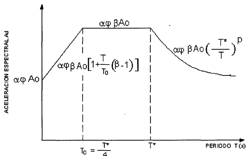
FIGURA 7.1 ESPECTRO DE RESPUESTA ELASTICO (R=1)
